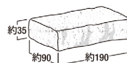
形状寸法図(mm)
