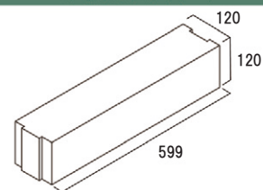
形状寸法図(mm)
