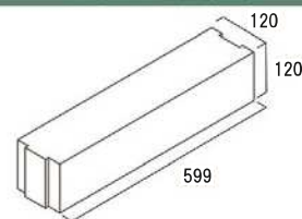
形状寸法図(mm)
